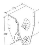
Suporte Mola Central CTA Facchini pino 60mm
