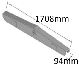
Balança Carreta Susp. Distanciada Randon 050
